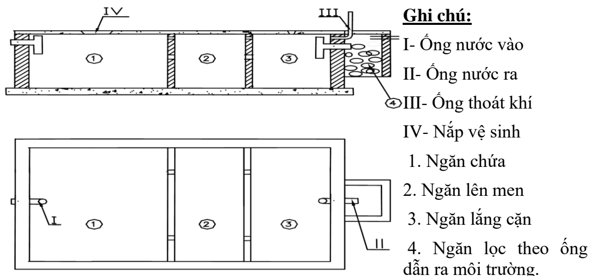
Hình 1.1. Mô hình bể tự hoại 3 ngăn
